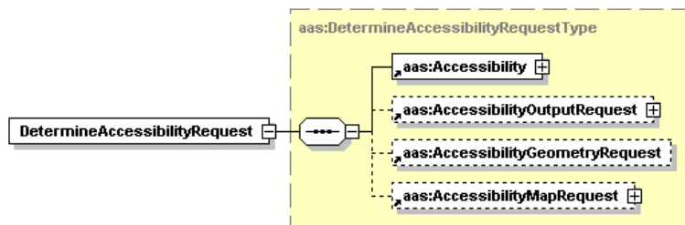
Abbildung 4: Schematische Darstellung des DetermineAccessibilityRequest-Schemas
