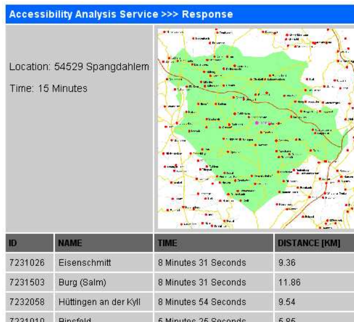
Abbildung 12: Prototyp der Web-Oberfläche für den AAS (Response)
