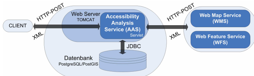
Abbildung 1: Architektur des Accessibility Analyse Service (AAS)
