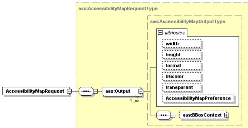
Abbildung 8: Schematische Darstellung des AccessibilityMapRequest-Schemas
